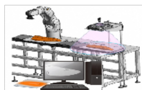
小骨自動除去ロボット
